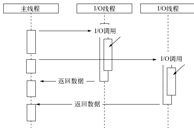
图3-9 异步I/O
