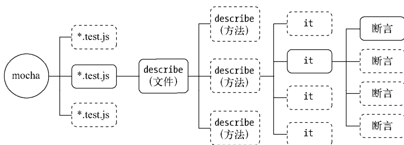
图10-1 BDD风格的组织示意图
