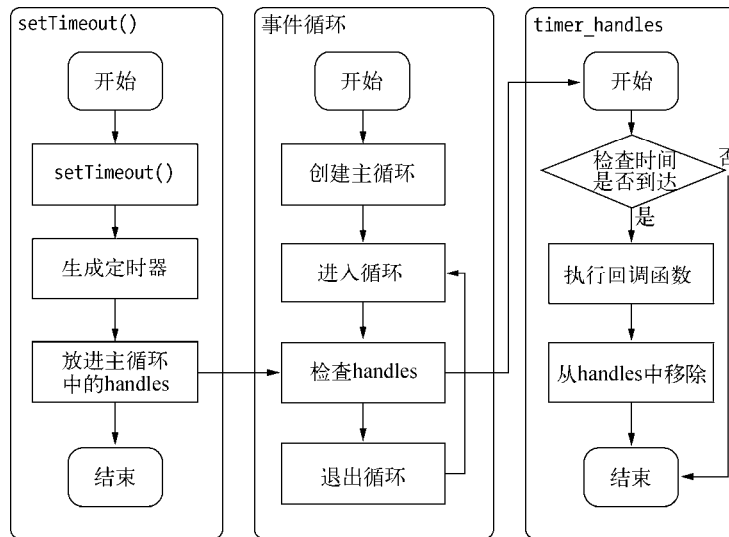
图3-14 setTimeout()的行为
