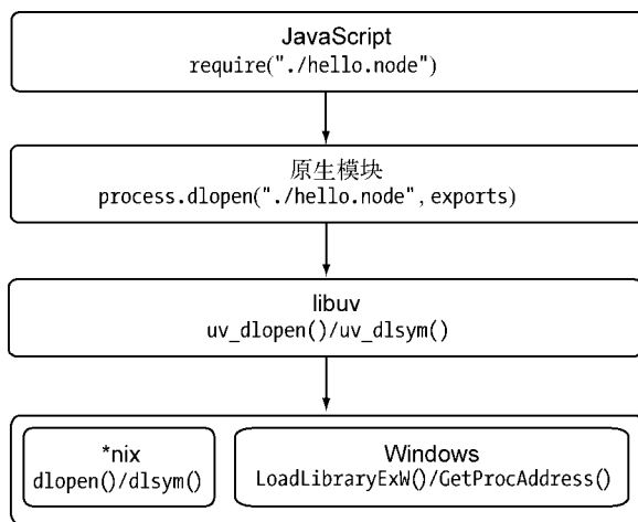
图2-7 require()引入.node文件的过程
