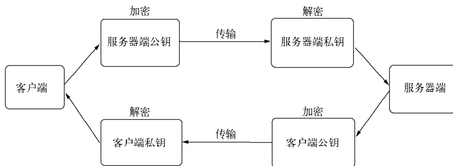
图7-8 客户端和服务器端交换密钥
