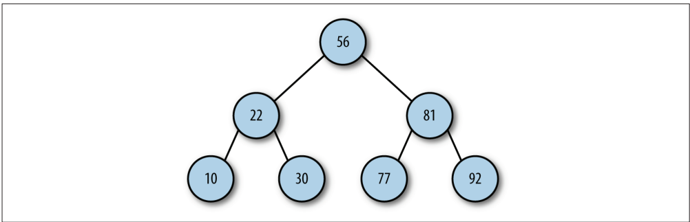
图 10-3：二叉树
