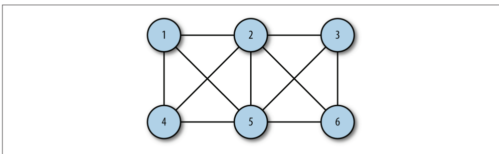
图 11-2: 无序图
