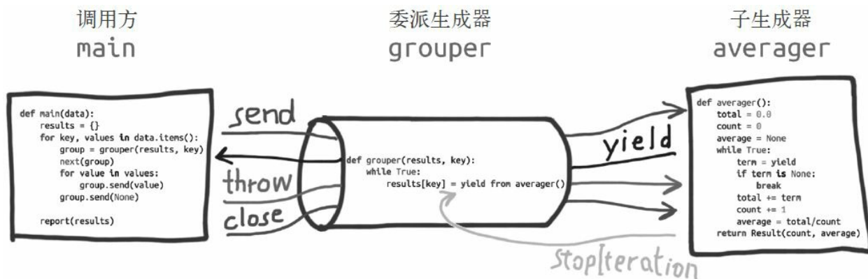
图 16-2: 委派生成器在 yield from 表达式处暂停时，调用方可以直接把数据发给子生成器，子生成器再把产出的值发给调用方。子生成器返回之后，解释器会抛出 StopIteration 异常，并把返回值附加到异常对象上，此时委派生成器会恢复
