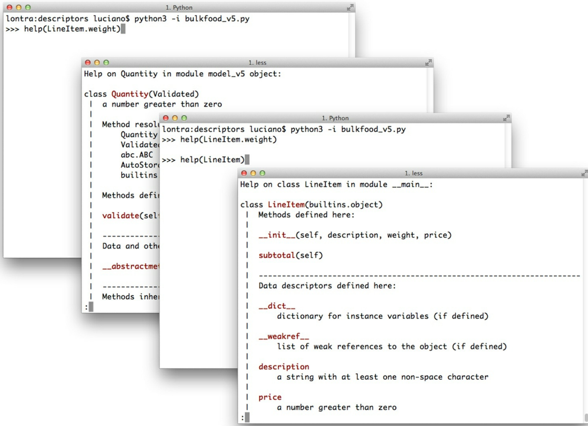
图 20-6: 在 Python 控制台中执行 help(LineItem.weight) 和 help(LineItem) 命令时的截图
