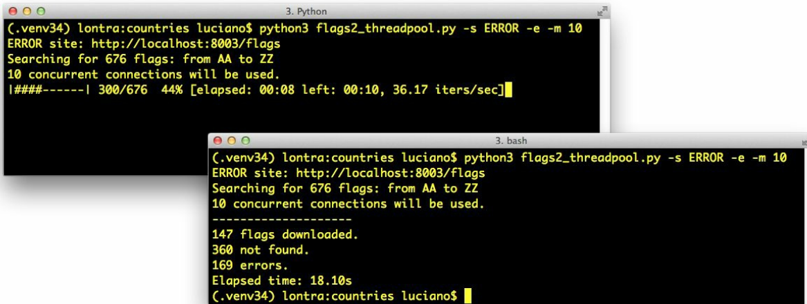
图 17-1：（左上） flags2_threadpool.py 运行中，显示着 tqdm 包生成的进度条；（右下）同一个终端窗口，脚本运行完毕后
