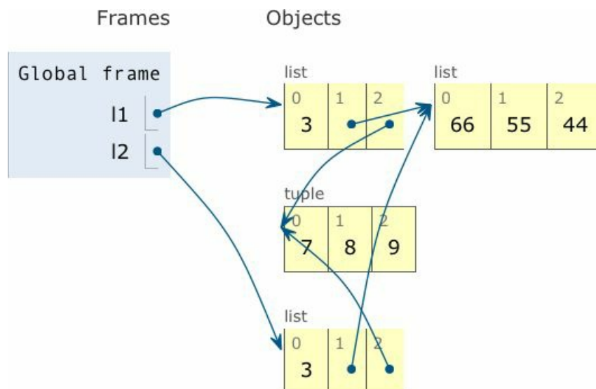
图 8-3: 示例 8-6 执行 l2 = list(l1) 赋值后的程序状态。11 和 12 指代不同的列表，但是二者引用同一个列表 [66, 55, 44] 和元组 (7, 8, 9) （图表由 Python Tutor 网站生成）
