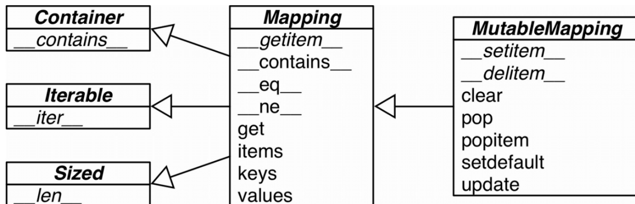
图 3-1: collections.abc 中的 MutableMapping 和它的超类的 UML 类图（箭头从子类指向超类，抽象类和抽象方法的名称以斜体显示）
