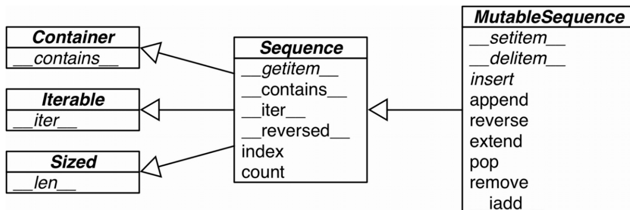
图 2-1: 这个 UML 类图列举了 collections.abc 中的几个类（超类在左边，箭头从
