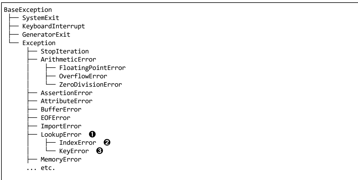
示例 11-10 异常类的部分层次结构
