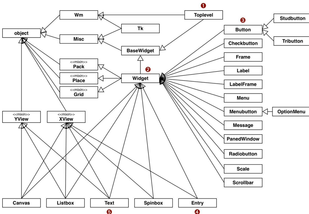
图 12-3: Tkinter GUI 类层次结构的 UML 简图；使用 <<mixin>> 标记的类通过多重继承为其他类提供具体方法
