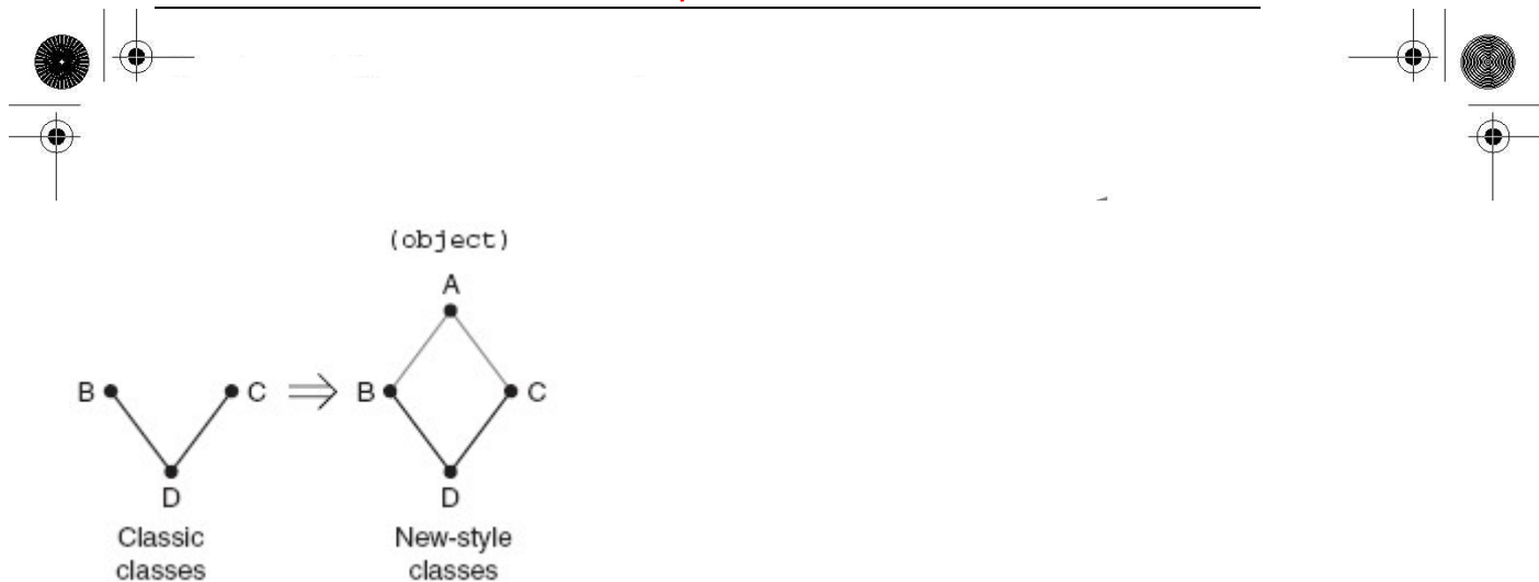
图 13.3 继承的问题是由于在新式类中，需要出现基类，这样就在继承结构中，形成了一个菱形。D 的实例上溯时，不应当错过 C，但不能两次上溯到 A（因为 B 和 C 都从 A 派生）。去读读 Guido van Rossum 的文章中有关“协作方法”的部分，可以得到更深地理解。
