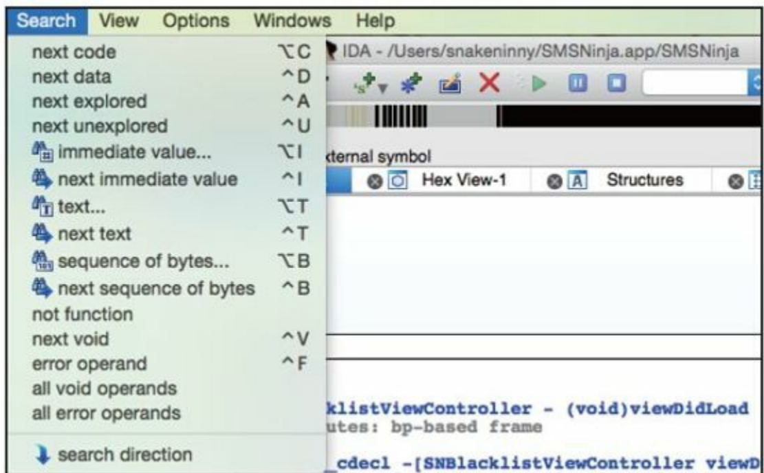
图3-44 在Main window里查找
