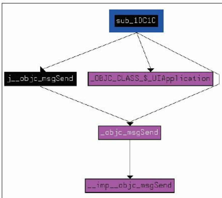
图3-42 查看sub_1DC1C显式引用的符号
