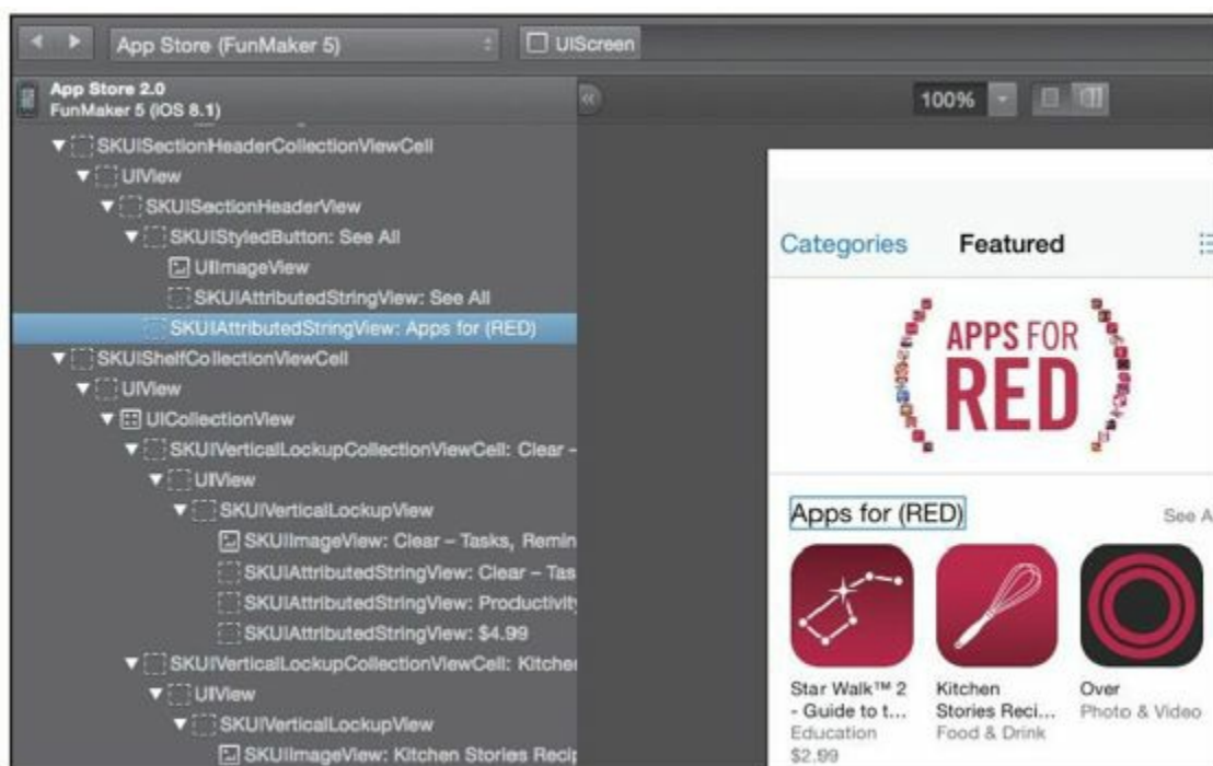
图3-16 用Reveal查看AppStore的UI布局
