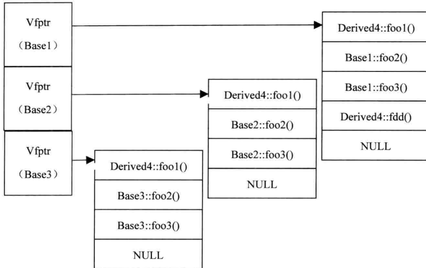
图 7.7 Derived4 虚函数表图
