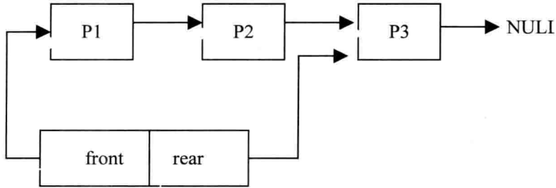
图 8.5 链表实现队列
