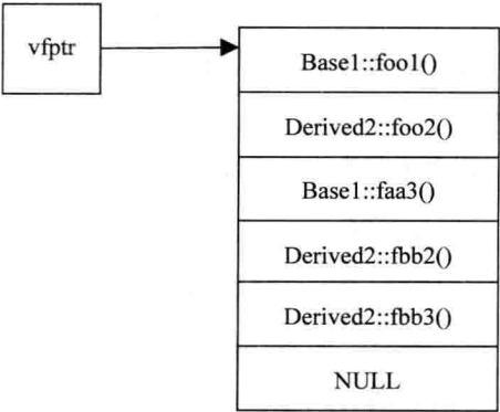
图 7.5 Derived2 虚函数表图
