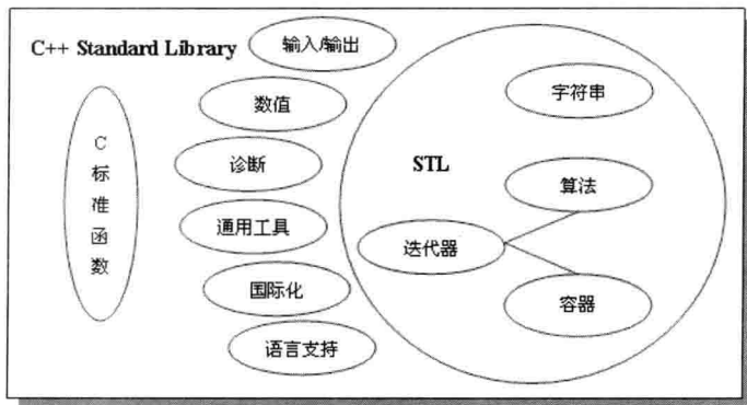
图 11.2 C++标准库中各组件关系
