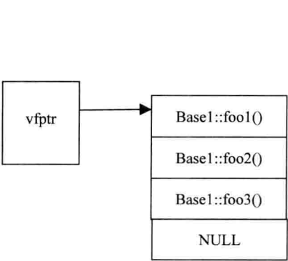
图 7.4 Derived1 虚函数表图
