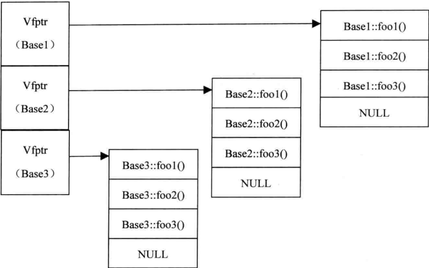
图 7.6 Derived3 虚函数表图
