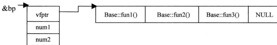
图 7.3 Base 虚函数表图
