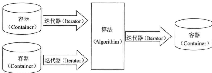
图 11.1 STL 组件之间的合作
