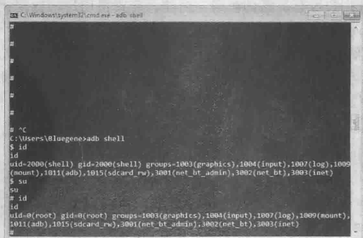
图 8.10 Android 设备 root 处理过程中的 Shell 控制台显示变化
