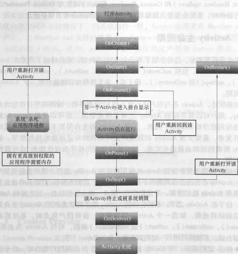
图 3.6 Activity 生命周期和回调函数
