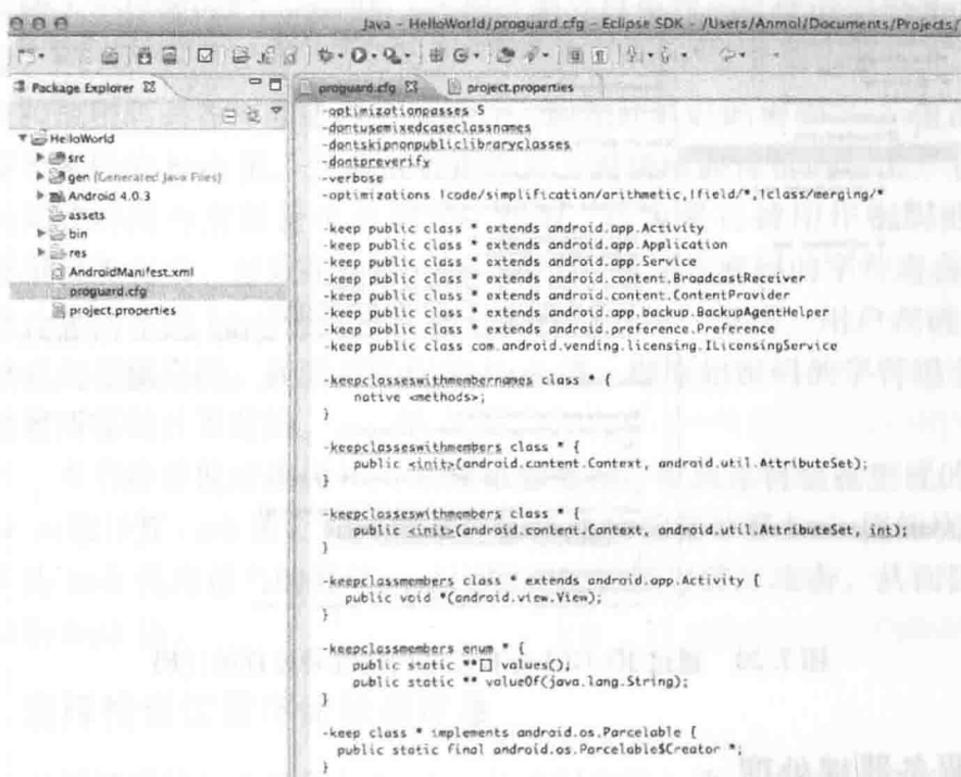
图 7.18 查看 Eclipse 开发环境下的 proguard. cfg 文件
