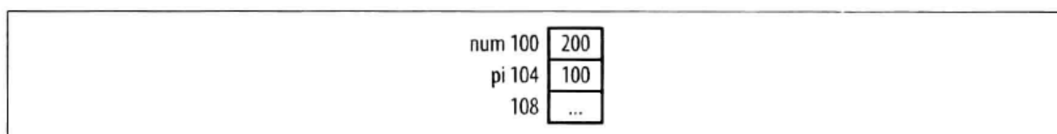
图 1-5：利用解引操作符给内存赋值
