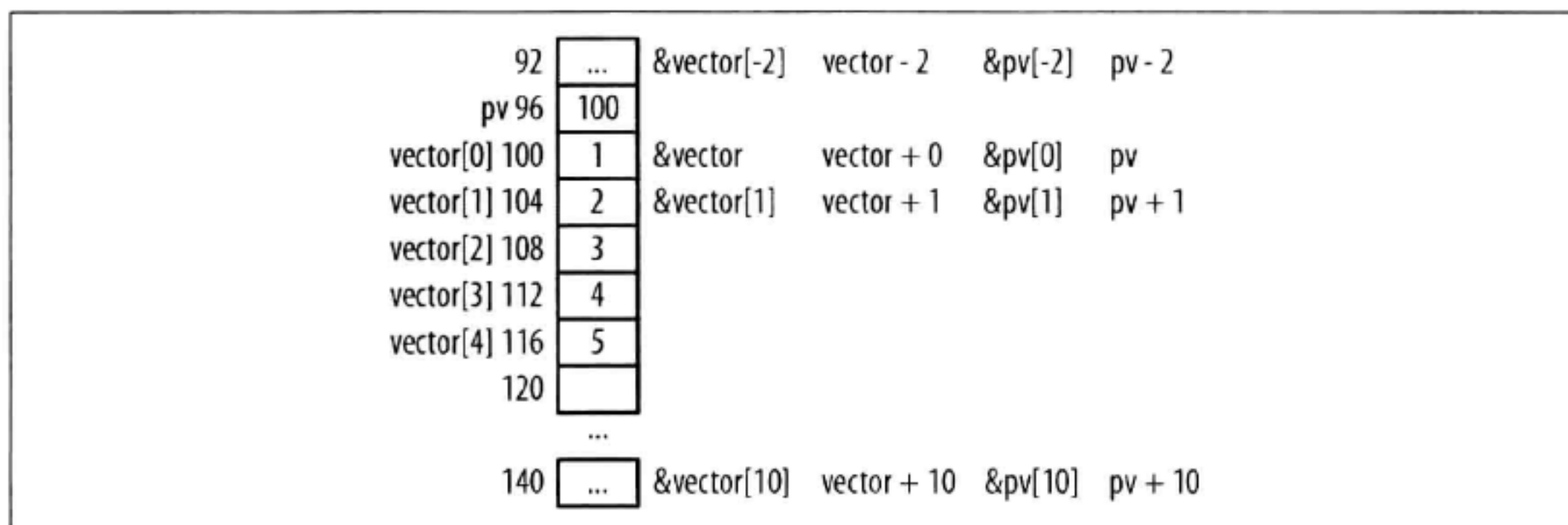
图 4-4：数组 / 指针表示法
