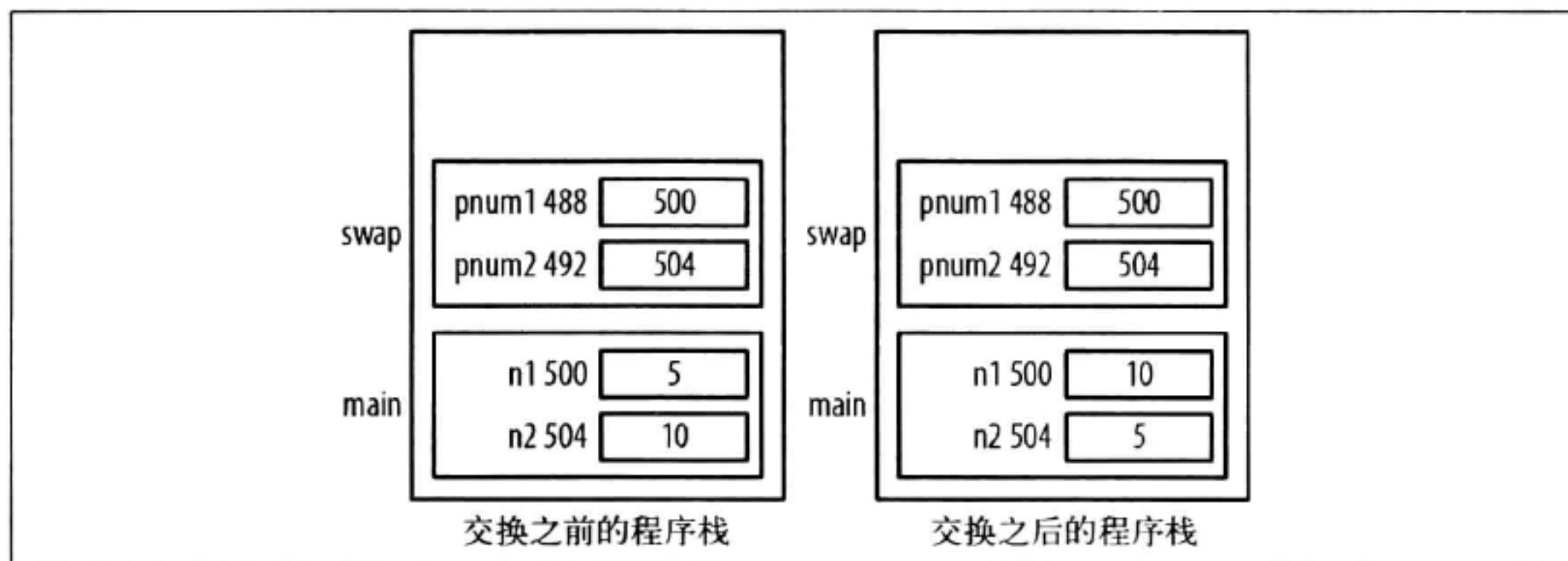
图 3-3：用指针实现交换
