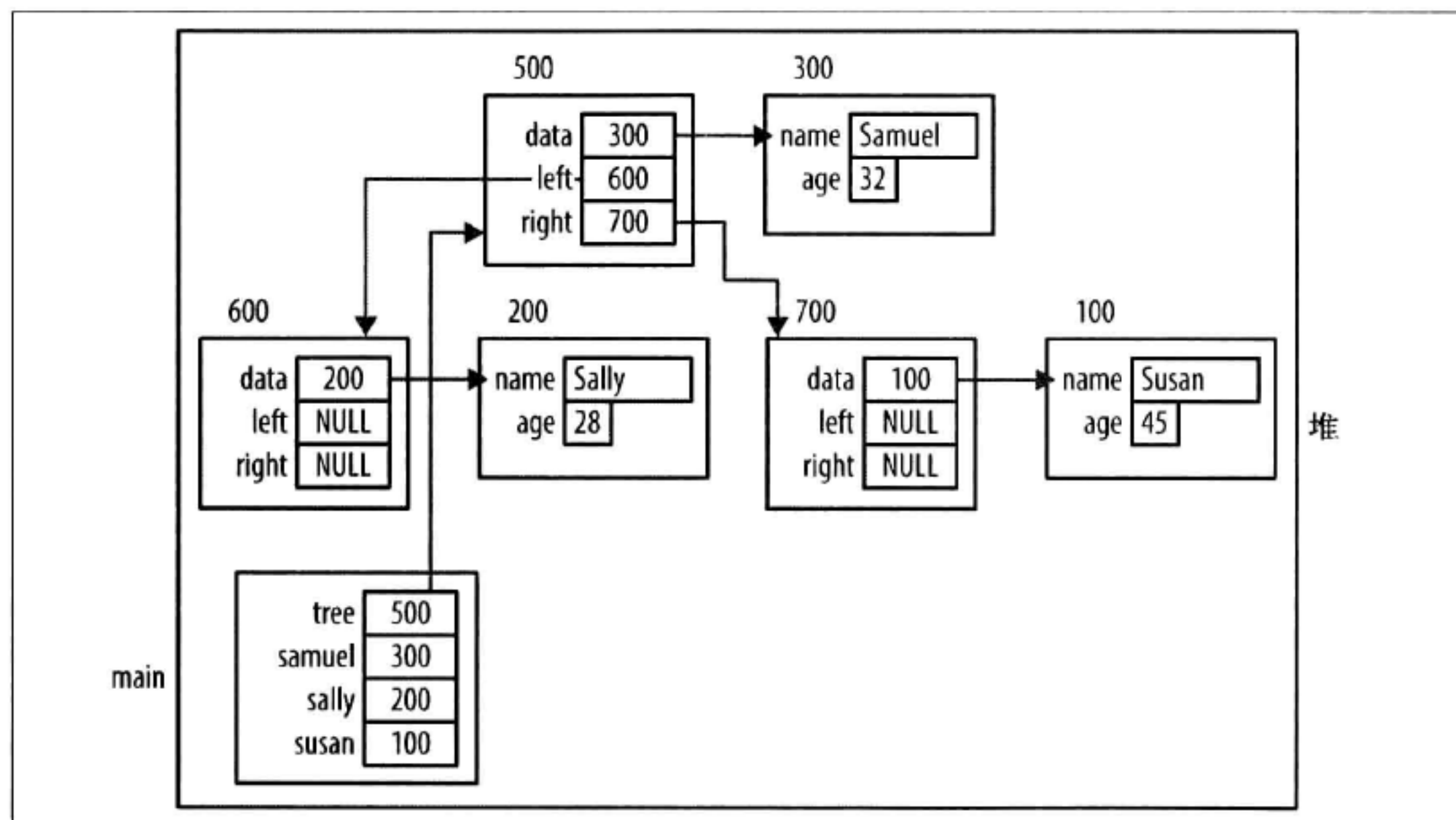
图 6-9: insertNode 函数
