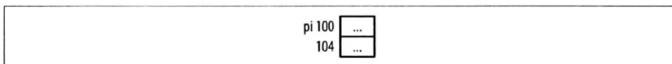
图 7-1：野指针
