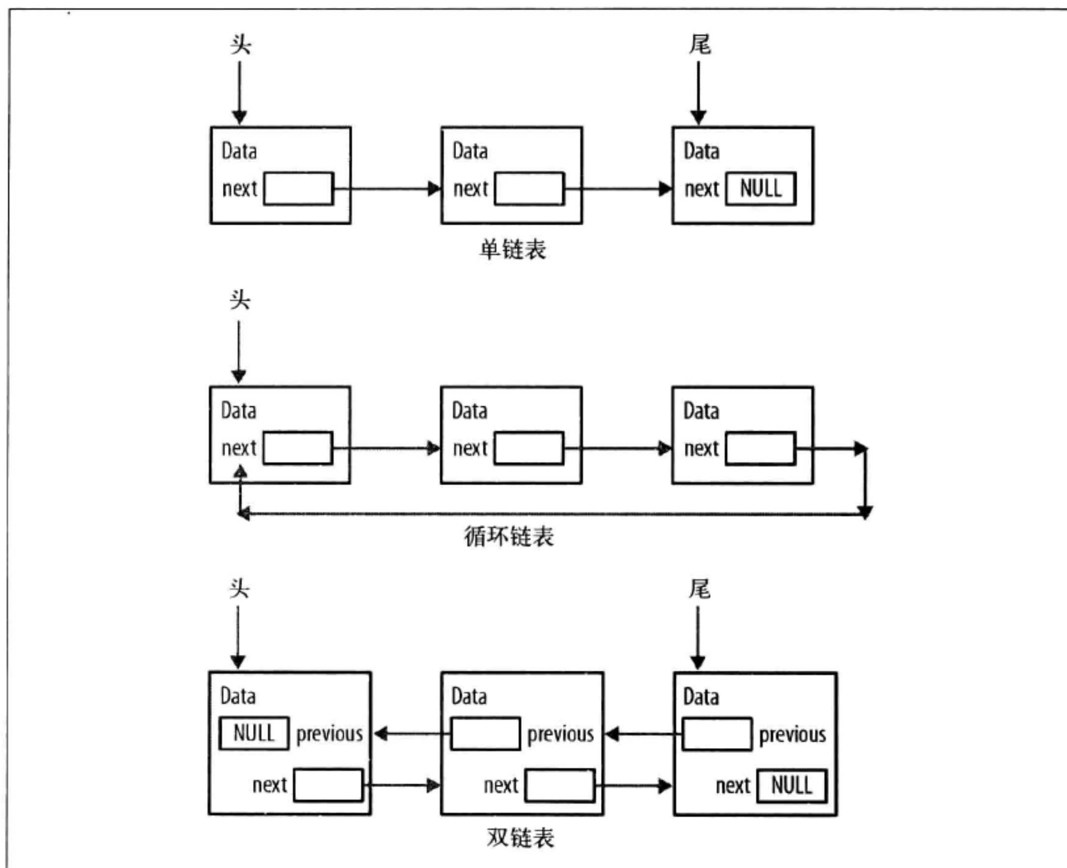
图 6-5：链表类型
