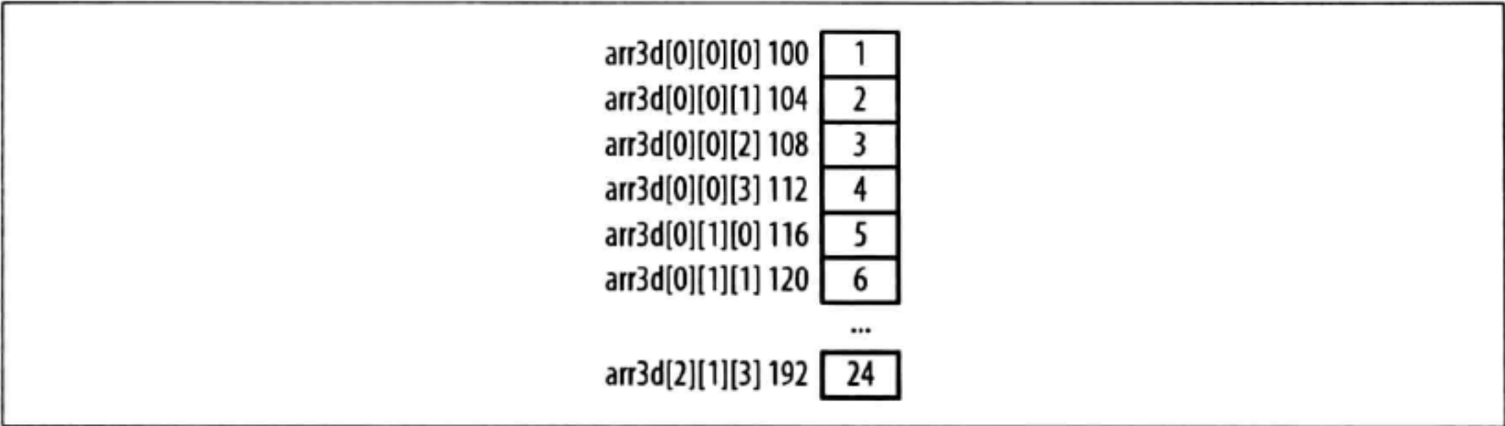
图 4-14：三维数组
