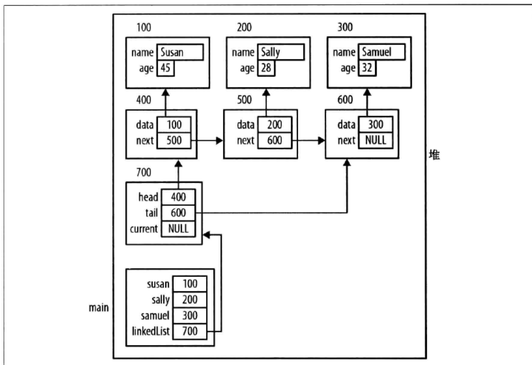
图 6-6: addHead 示例
