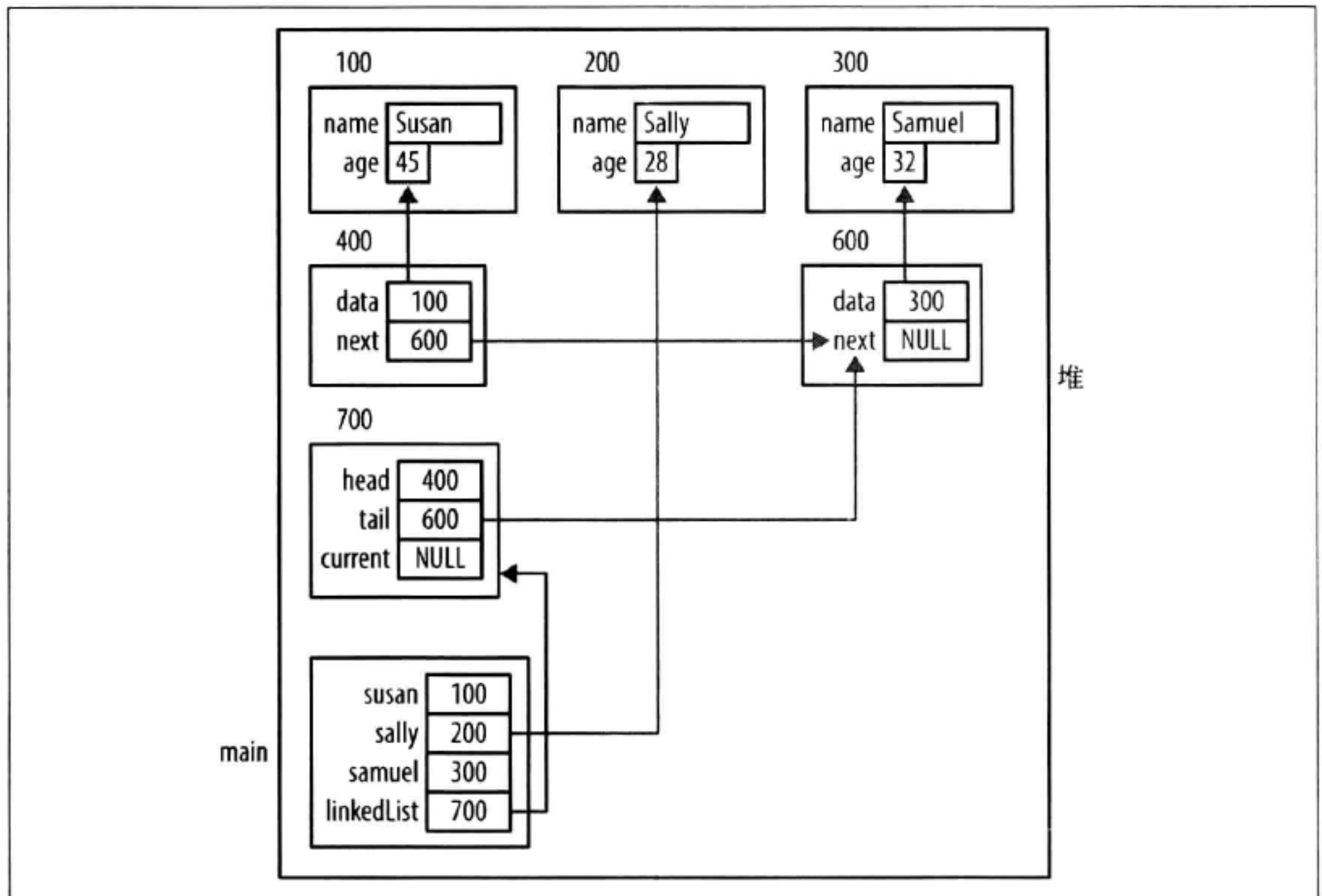
图 6-7：删除示例
