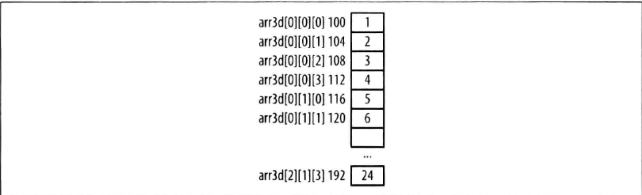
图 4-3：三维数组
