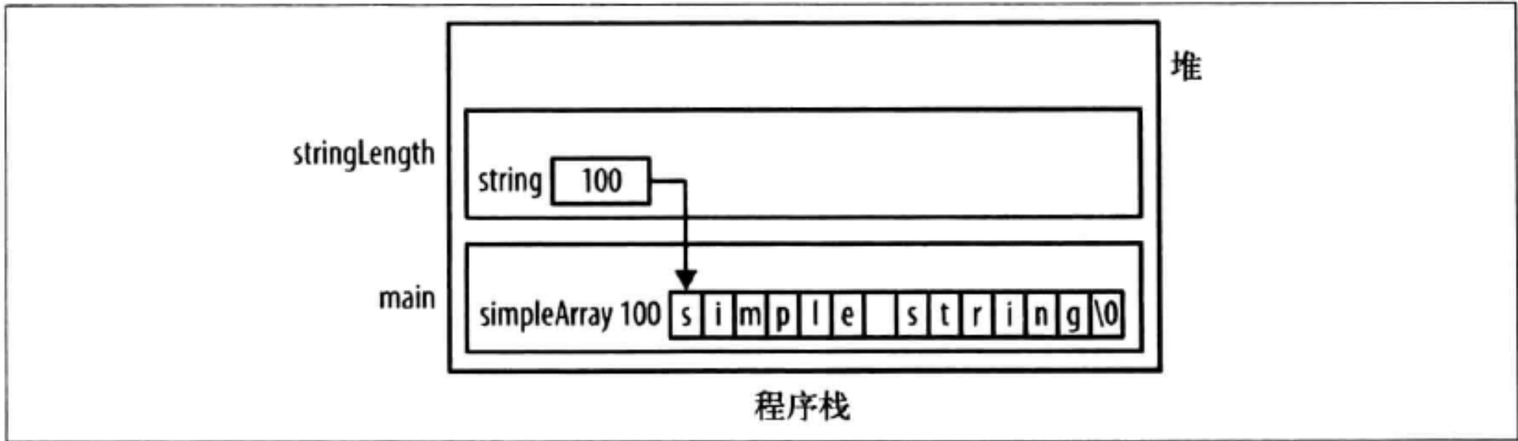
图 5-12：传递字符串
