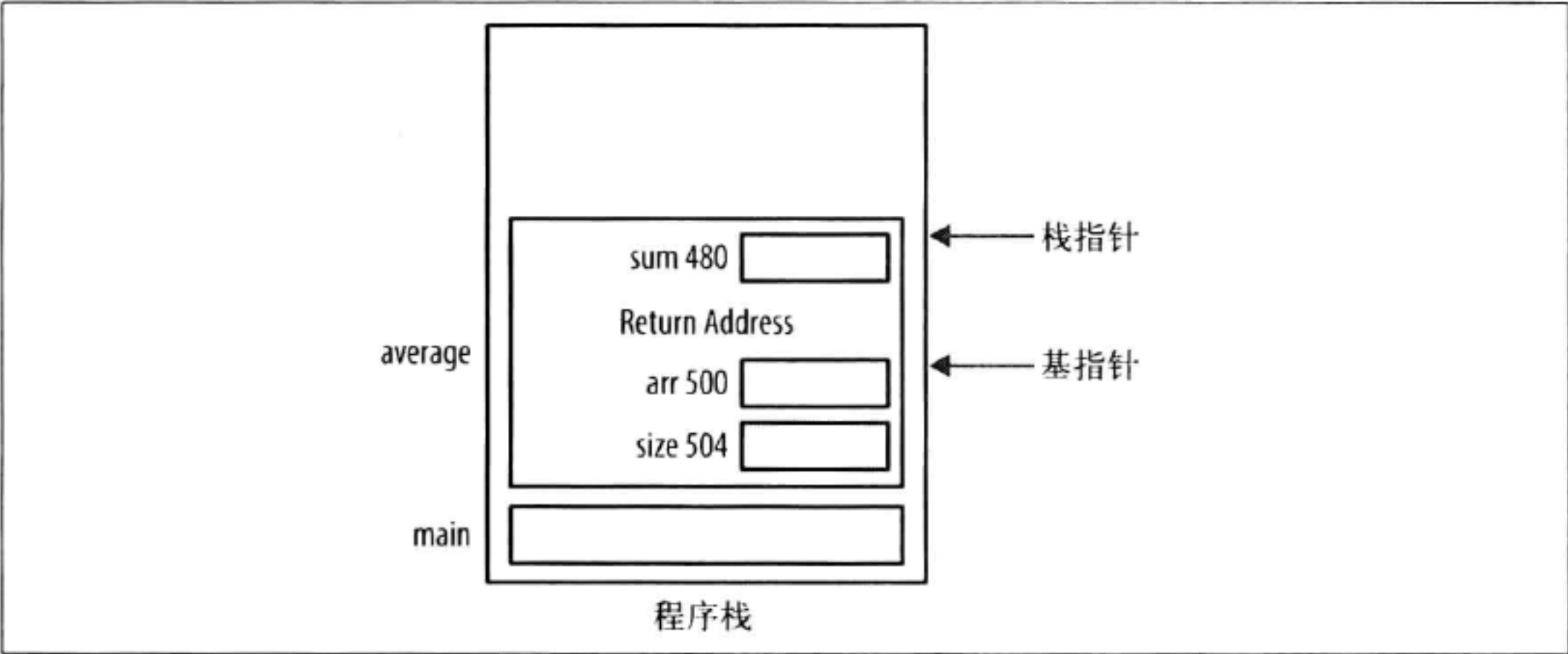
图 3-2：栈帧示例
