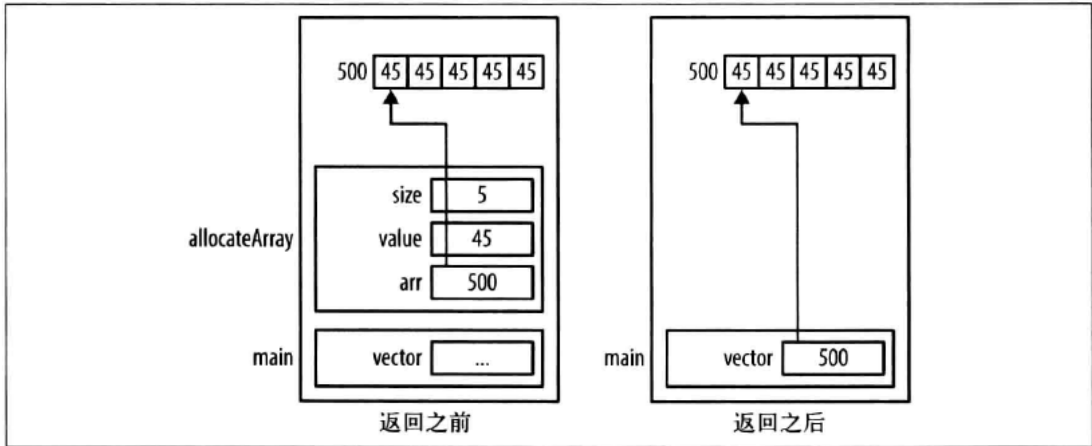
图 3-5：返回指针
