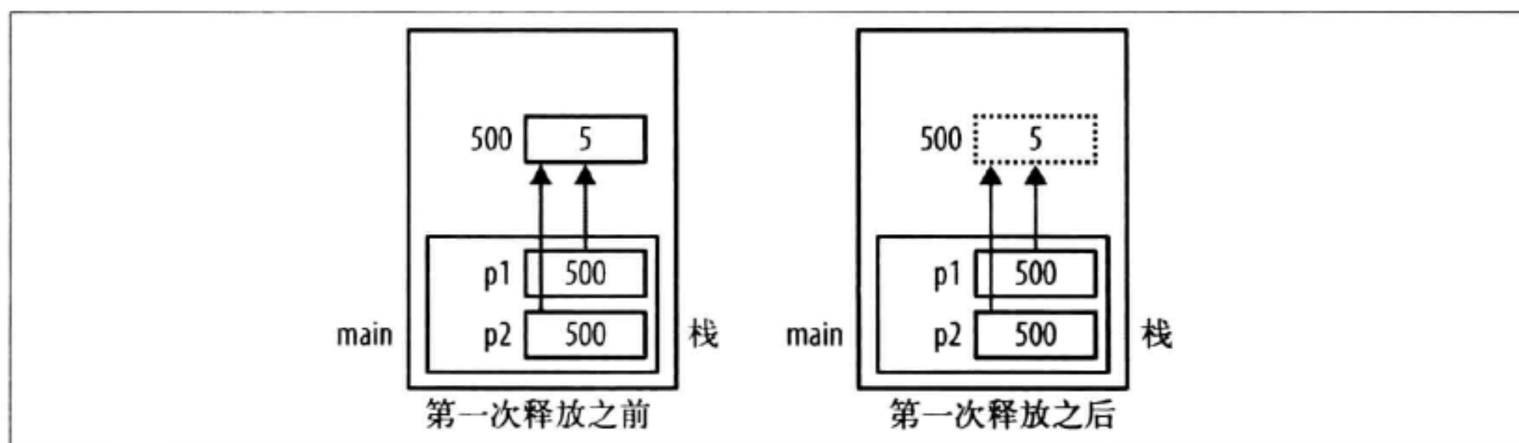
图 2-10：重复释放
