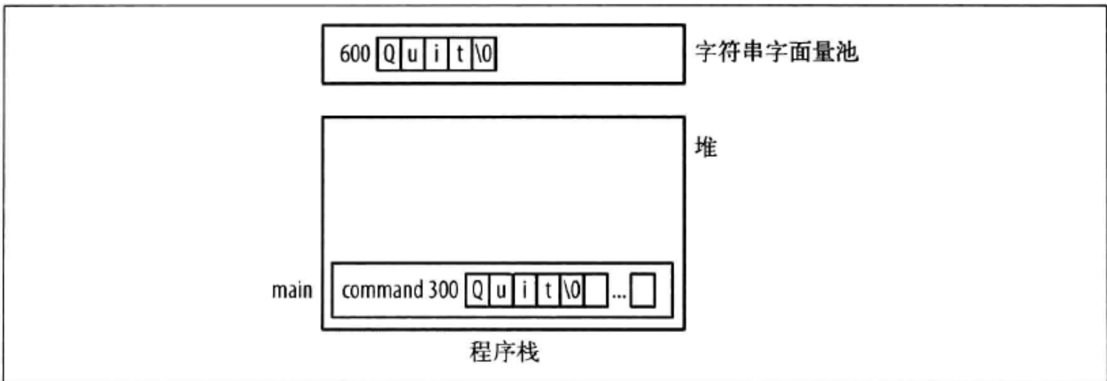
图 5-6: strcmp 示例
