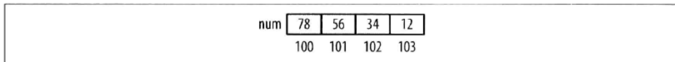
图 8-4: 字节序示例
