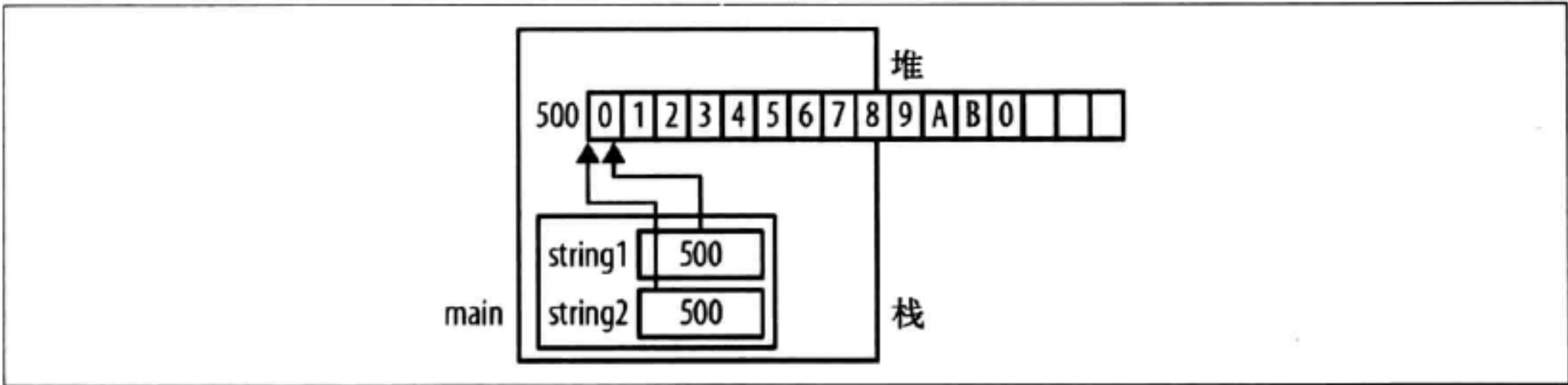
图 2-6: realloc 示例
