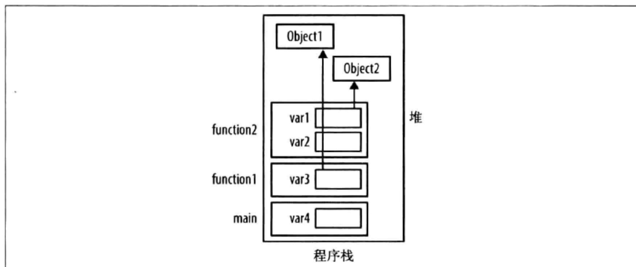
图 3-1：栈和堆
