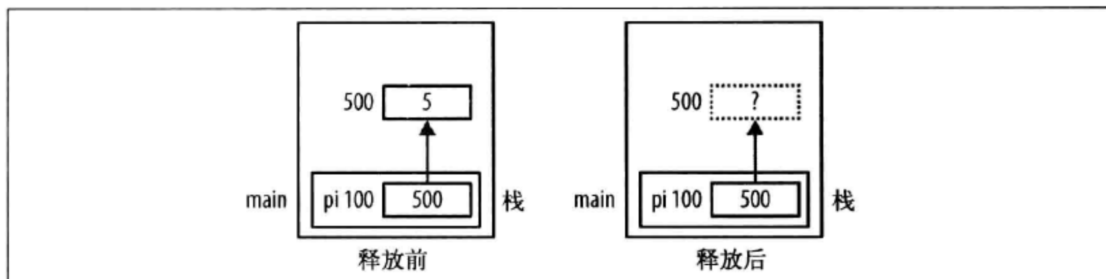
图 2-11：迷途指针
