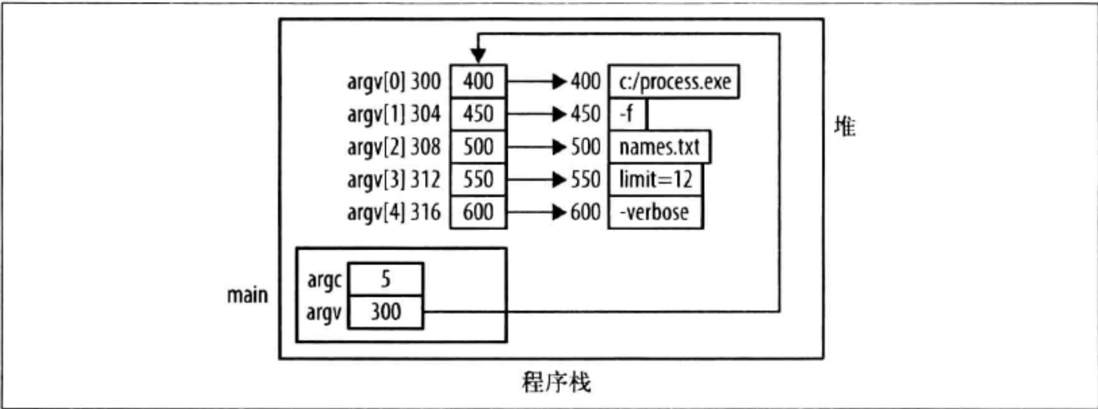
图 5-13：使用 argc/argv
