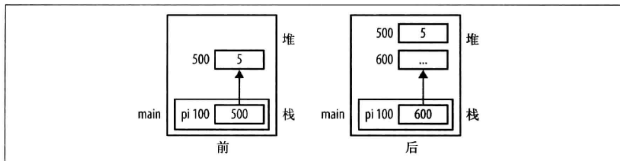
图 2-3：丢失地址
