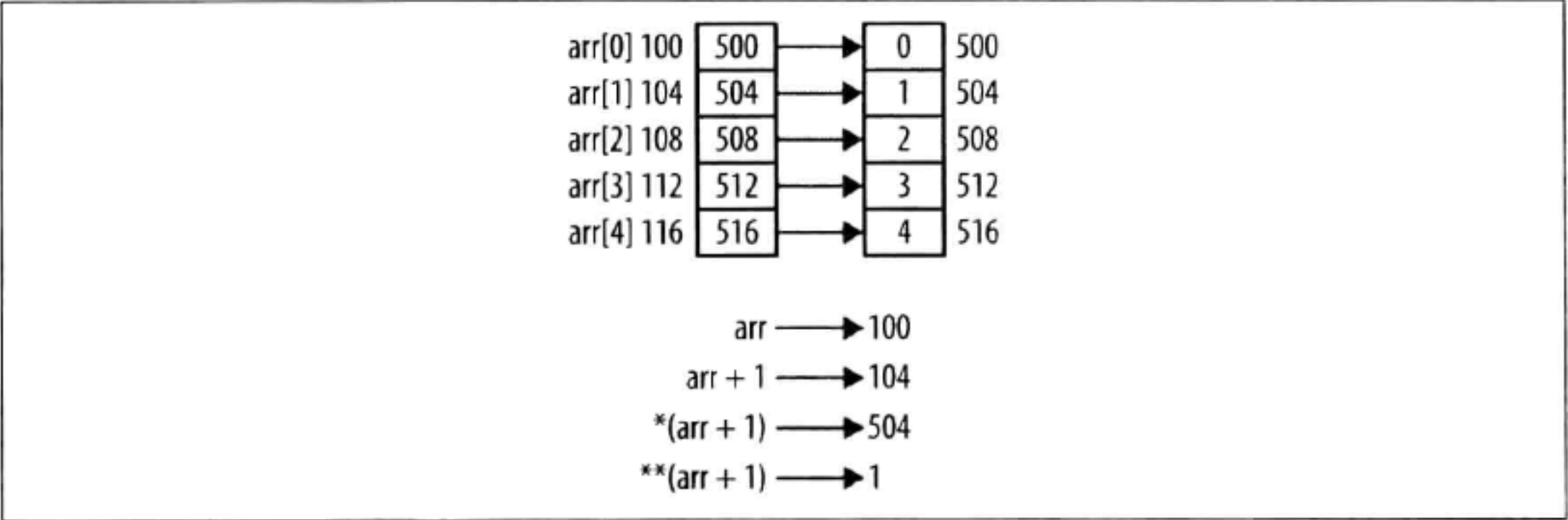
图 4-9：指针数组
