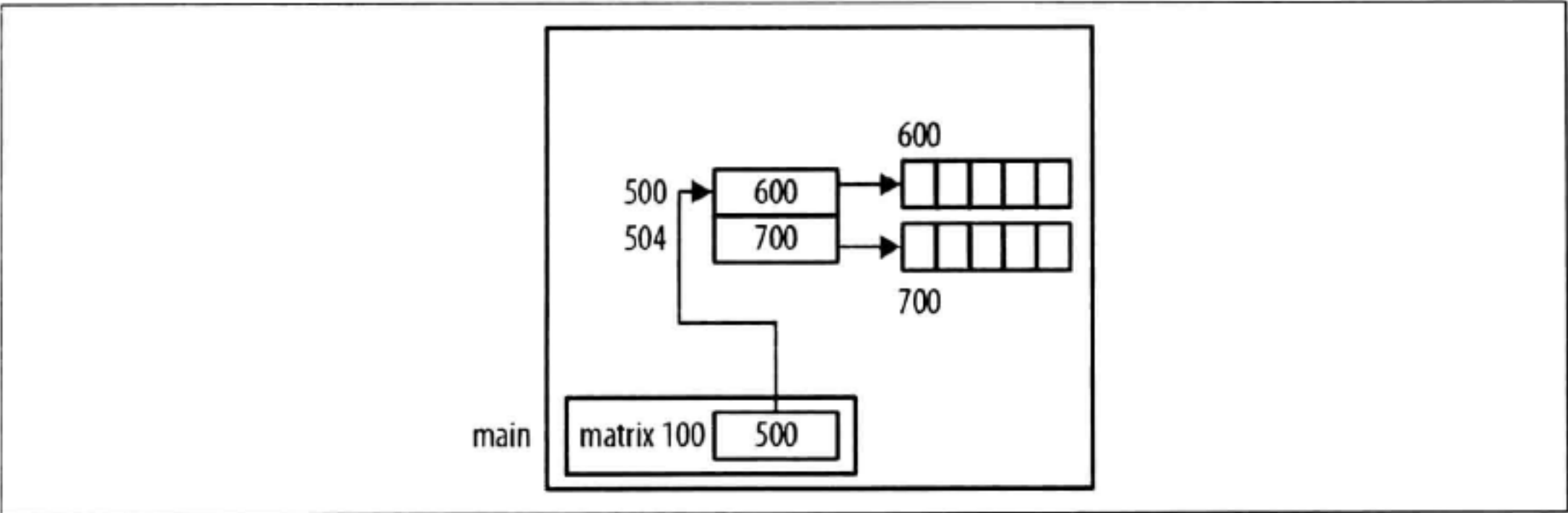
图 4-15：不连续分配
