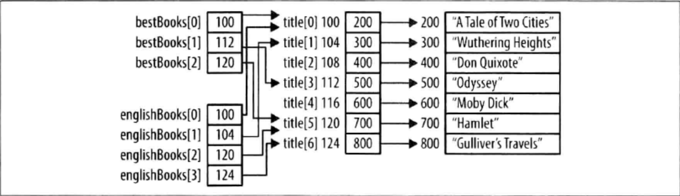
图 1-10：指针的指针
