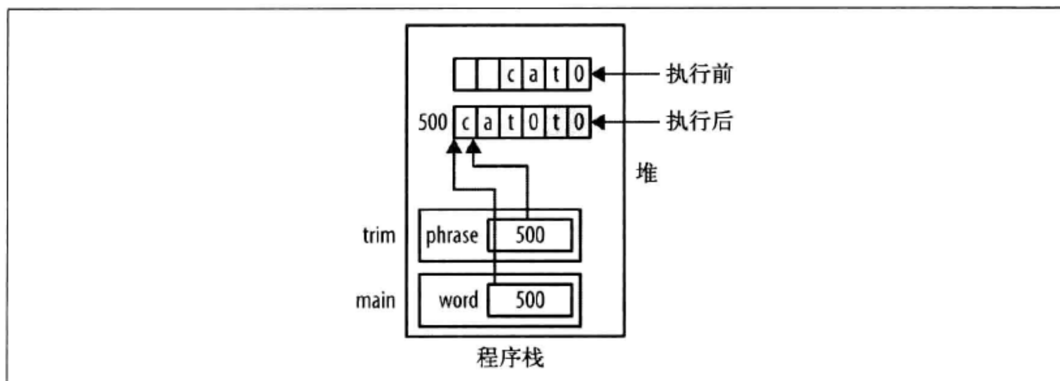
图 4-7: realloc 示例
