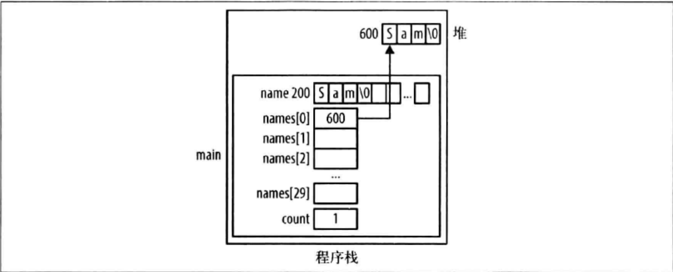
图 5-7：复制字符串
