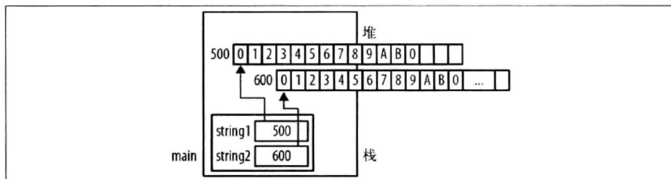
图 2-7：分配额外内存
