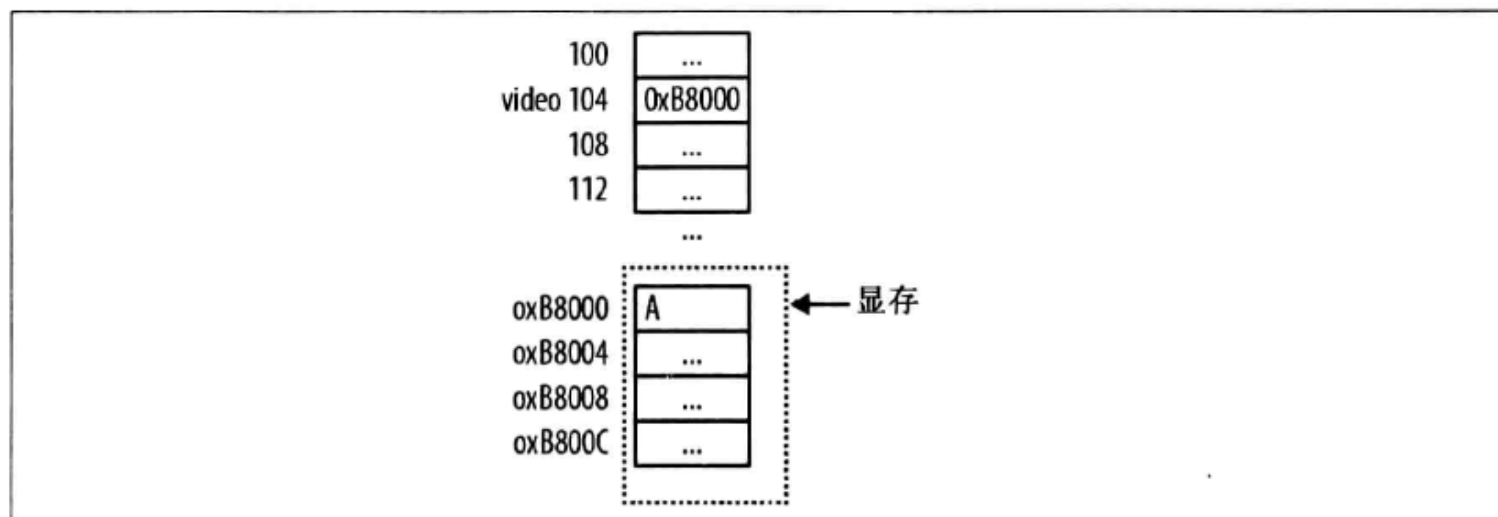
图 8-2：在 PC 上寻址显存
