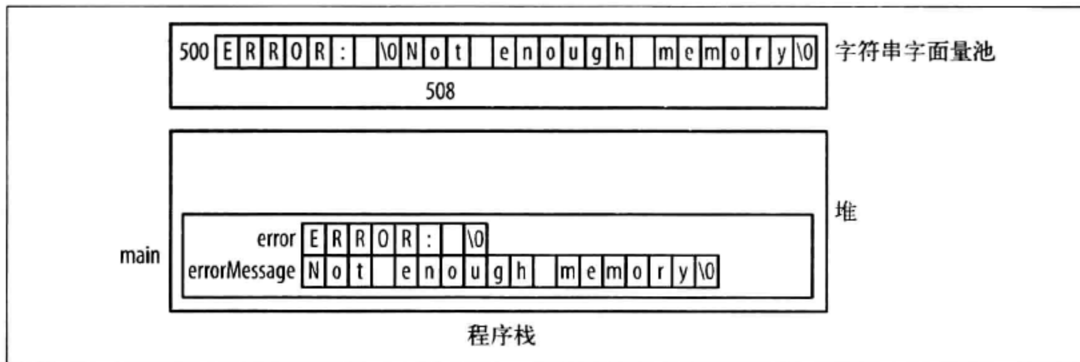
图 5-11: 覆写栈帧
