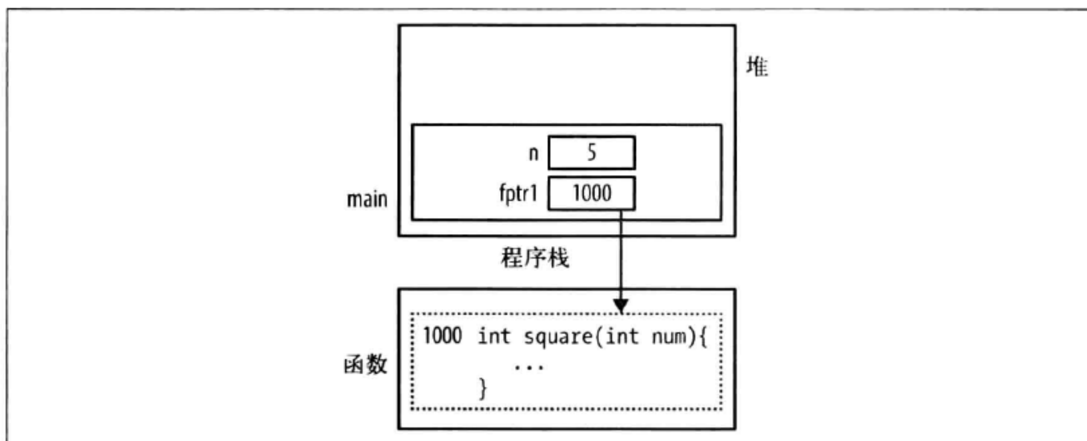
图 3-10：函数的位置
