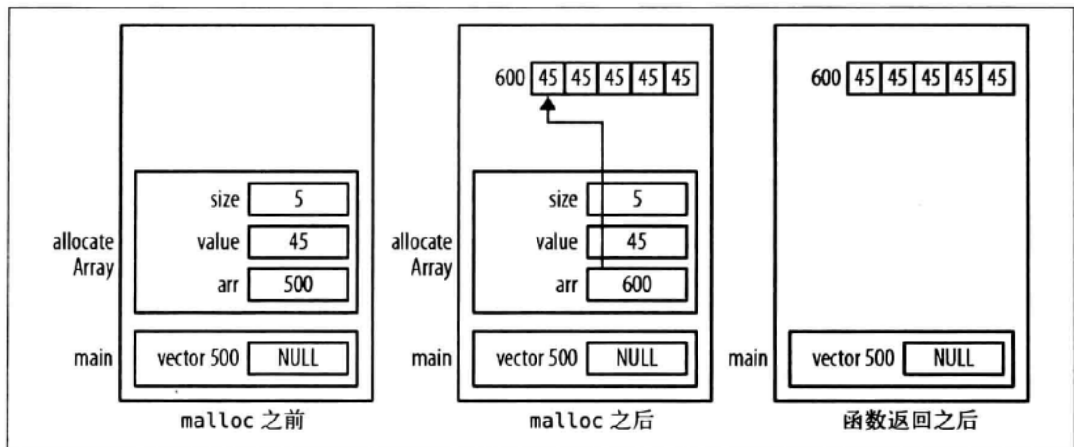
图 3-8: 传递指针
