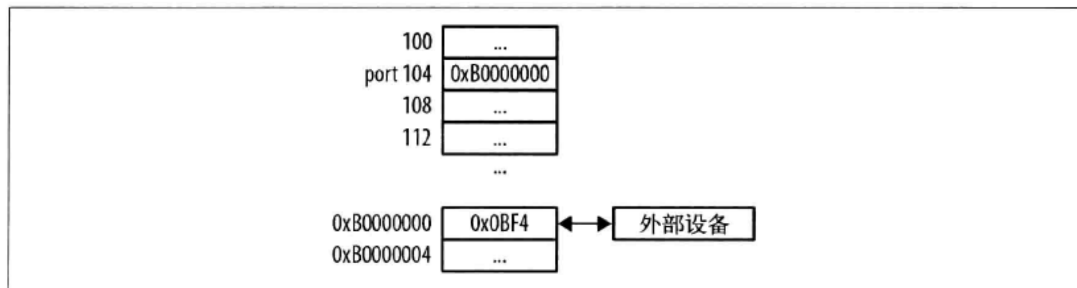
图 8-3: 访问端口
