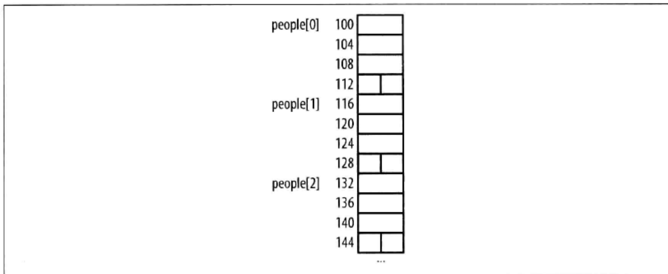
图 6-1: AlternatePerson 的数组
