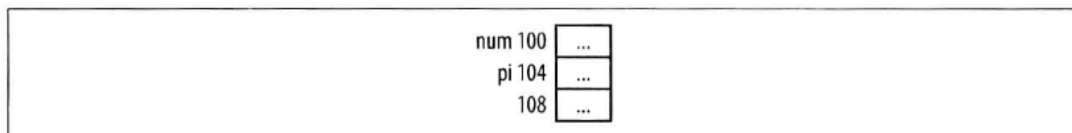
图 1-2: 内存图解
