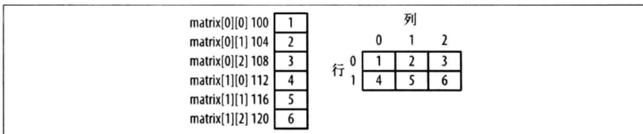
图 4-2：二维数组
