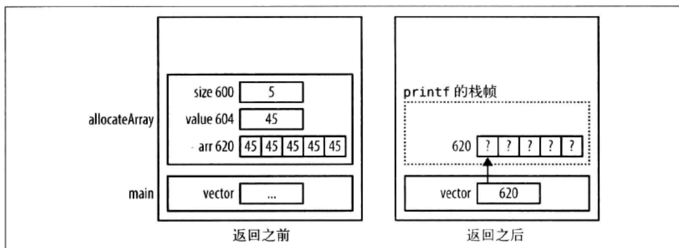
图 3-6：返回局部数据的指针
