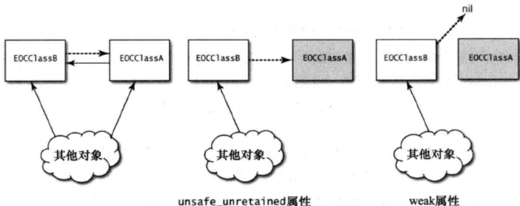
图 5-6 unsafe_unretained 与 weak 属性，在其所指的对象回收以后表现出来的行为不同
