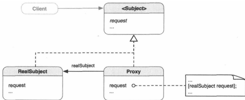
图22-1 代理模式的类图
