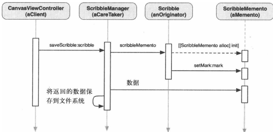
图2-11 说明Scribble的状态如何保存为ScribbleMemento对象的时序图
