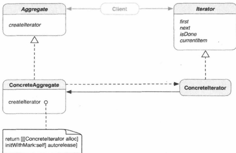
图14-2 更进一步表示抽象列表与迭代器之间关系的类图
