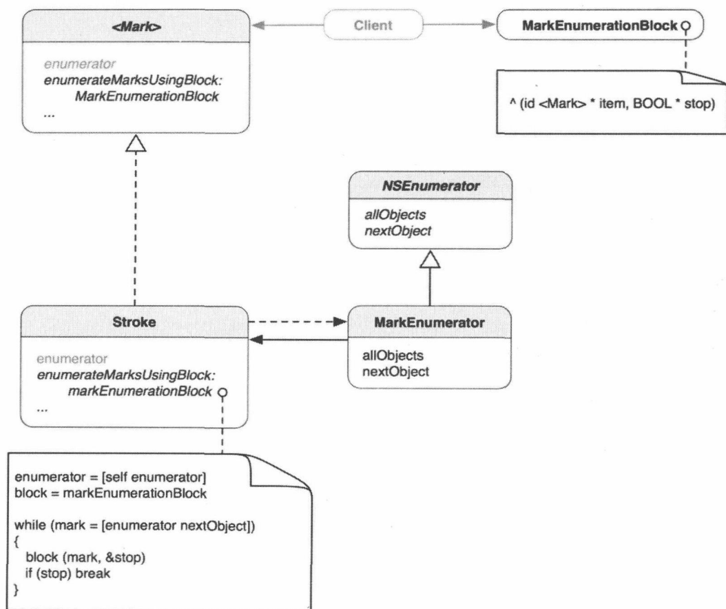
图14-4 MarkEnumerator和Stroke的修改版本的类图。通过引入MarkEnumerationBlock实现了内部迭代器
