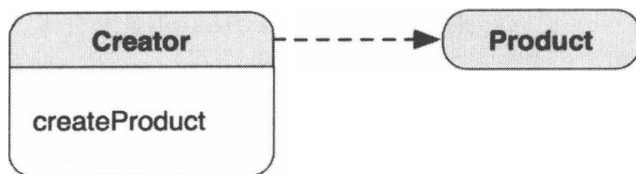
图1-5 一个类实例化另一个类
