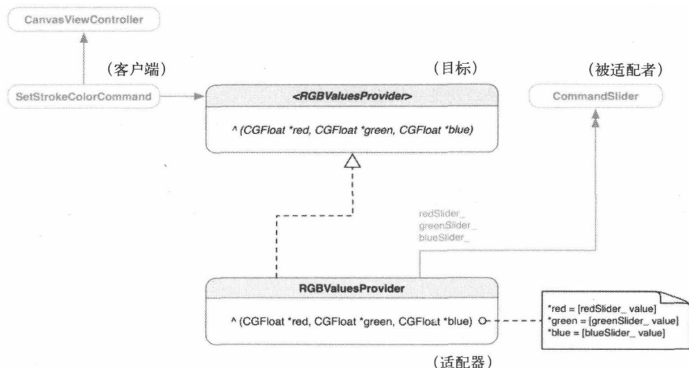
图8-4 使用对象组合适配UISlider实现RGBValuesProvider块作为StrokeColorCommand的对象适配器的类图
