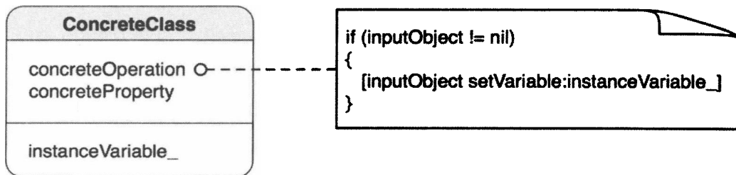
图1-9 伪代码笔记
