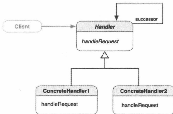
图17-1 责任链模式的类图
