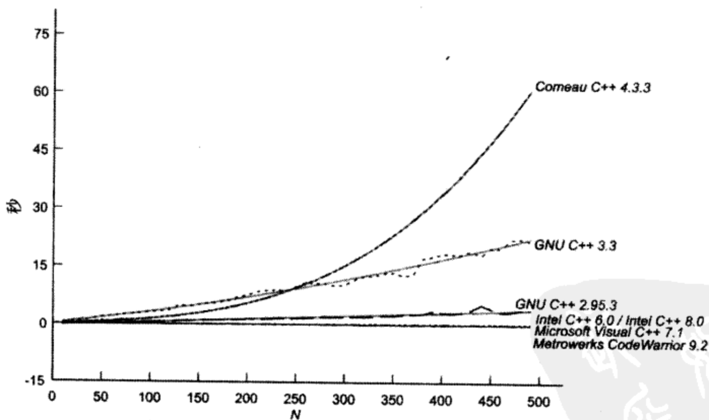
图C.11 递归实例化时间 vs. 实参嵌套深度 (Argument Nesting Depth)
