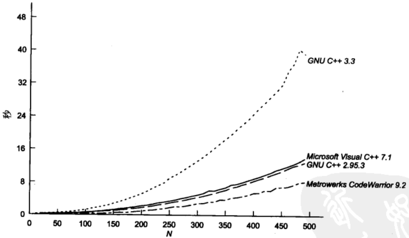
图C.6 时间 vs. 嵌套深度
