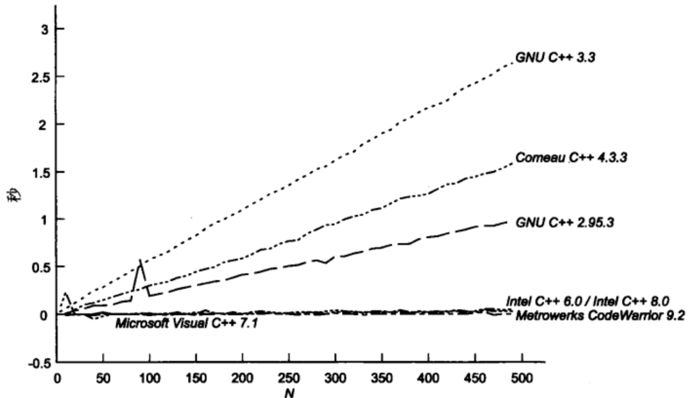
图C.9 递归实例化时间与实参的元数
