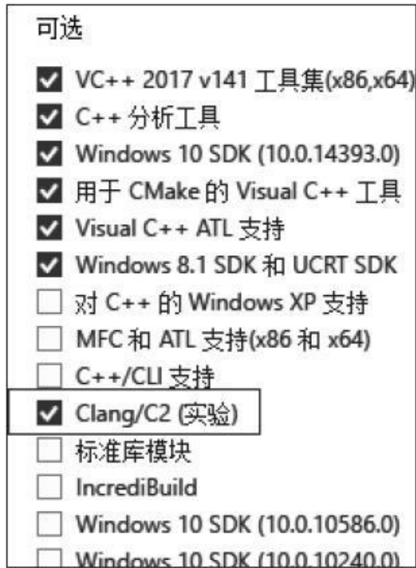
图3-1 Visual Studio Community安装界面
